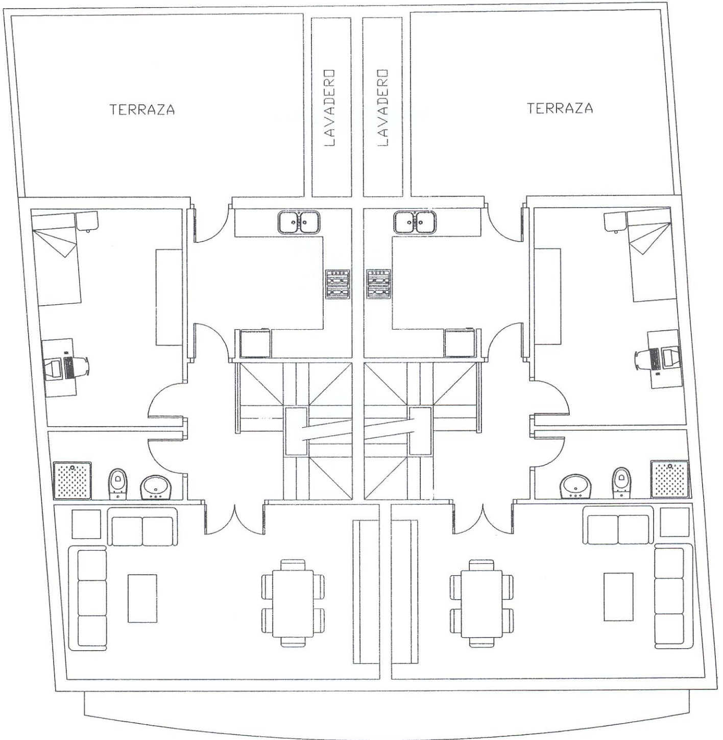
PLANTA PRIMERA
